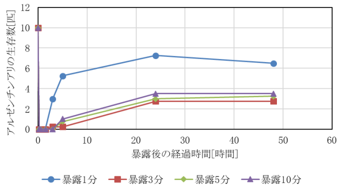
図2 暴露耐性試験結果 (ARINIX® I )
