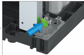
ストッパー閉状態(オートロック機能付) ※上下のレバーを同時に押し込むとストッパーが開く。
